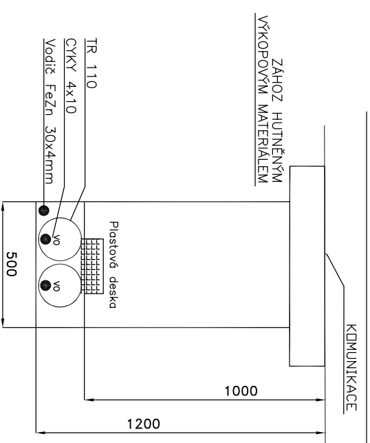
ŘEZ D-D'
