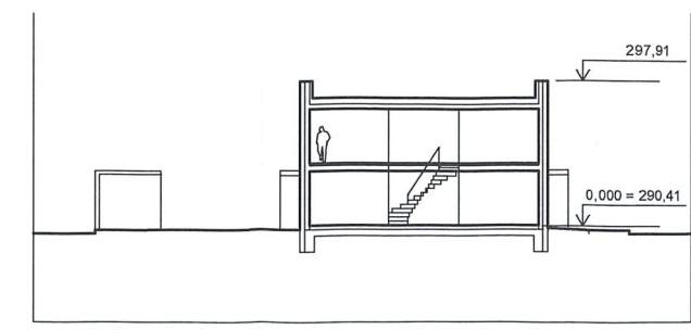
ŘEZ BEZ PODKROVÍ
