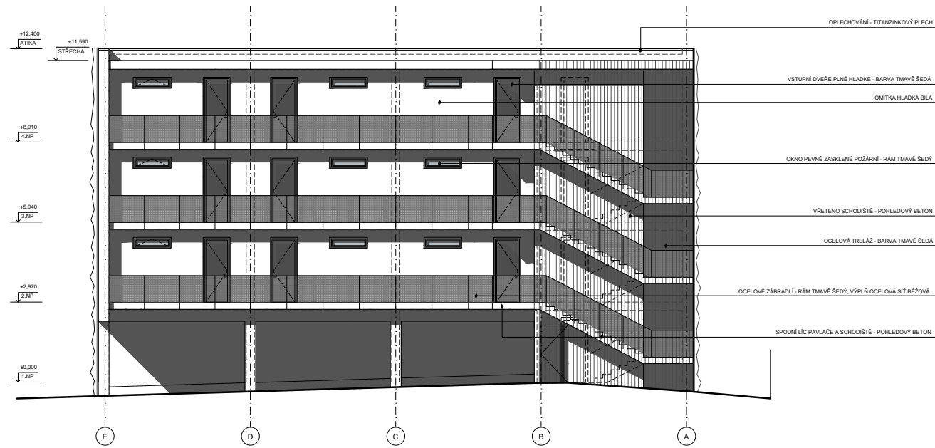
pohled severovýchodní
