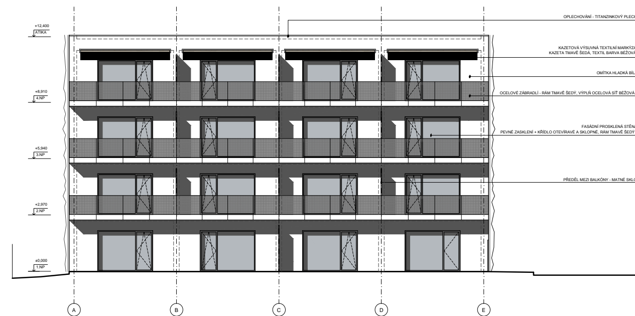
pohled jihozápadní
