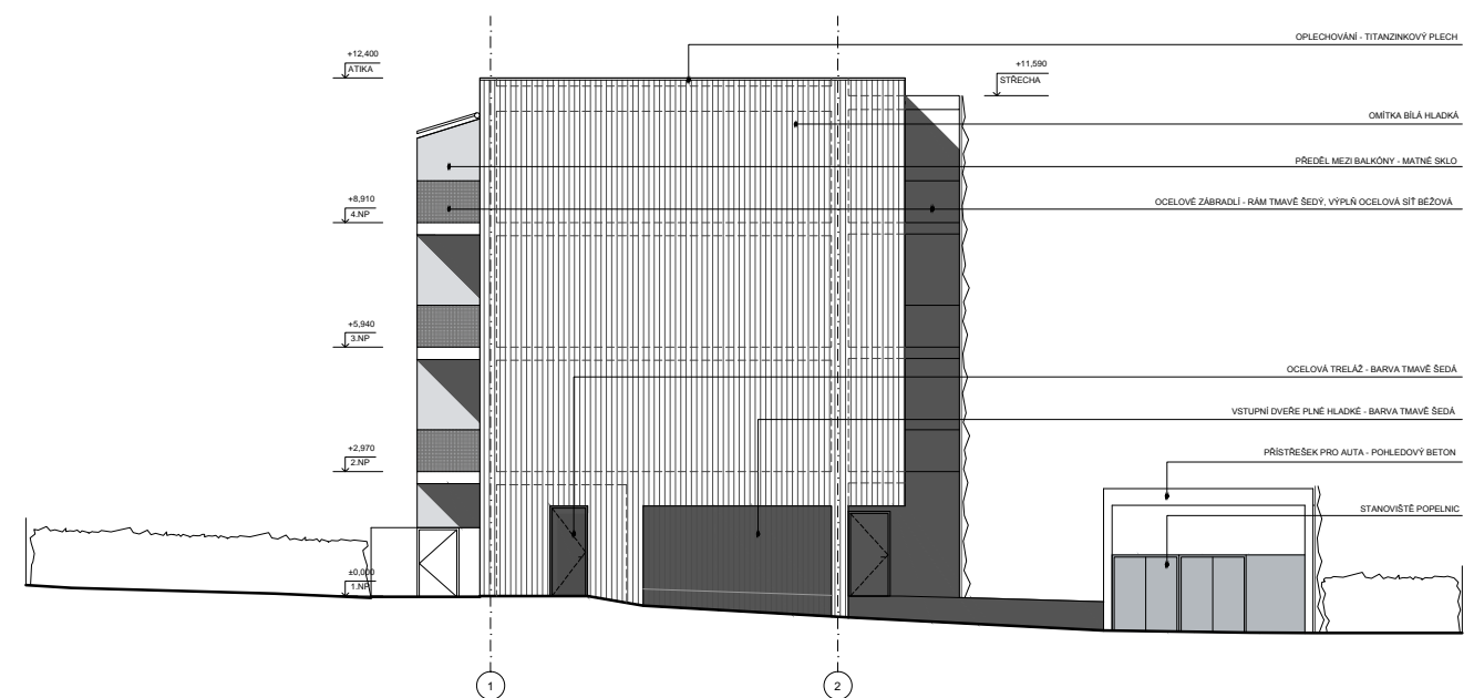
pohled jihovýchodní
