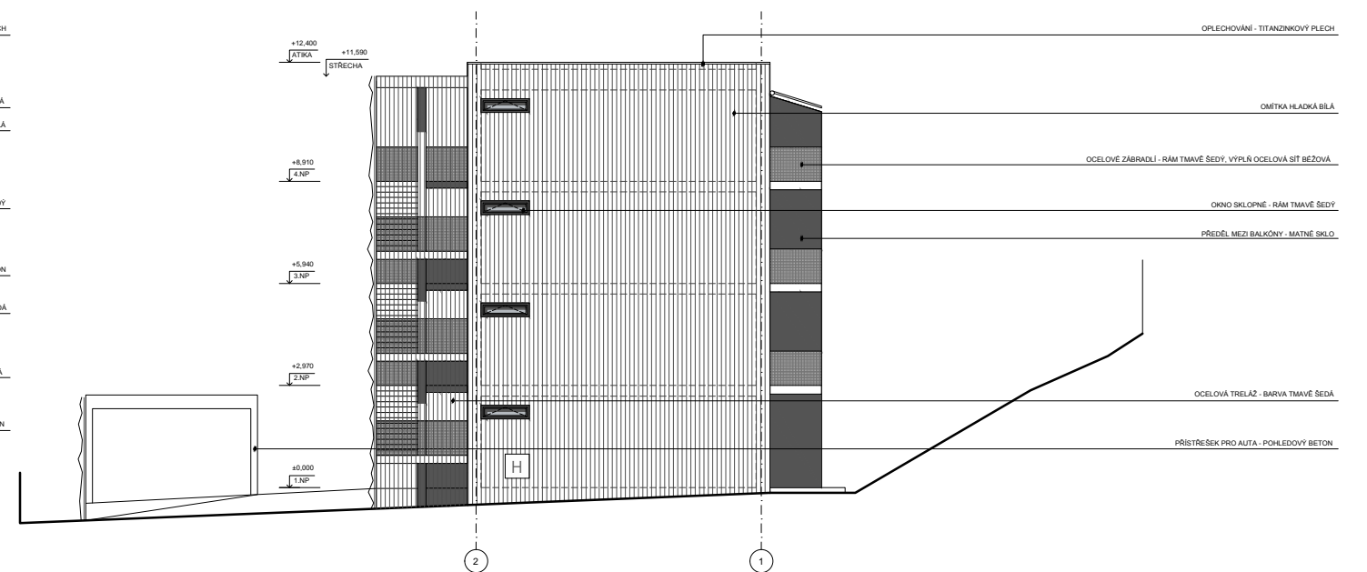
pohled severozápadní
