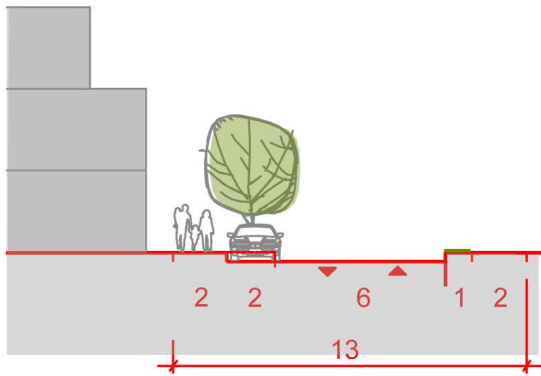
řez 1-1
