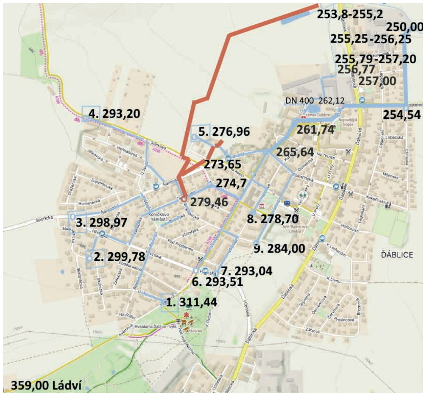
Významnější dešťové stoky západní a střední části Ďáblic s vyznačením výšky dna jejich začátků, resp. křížení dle Digitální technické mapy Prahy (1.–4. procházejí křížením Brigádnická–Čenkovská 279,46; 1.–9. procházejí křížením Květnová – Ke Štamberku 265,64) a výšky dna – maximální hladiny poldru, resp. budoucí vodoteče mezi Statkem a poldrem dle dokumentace Obytný soubor Statek Ďáblice – 1. etapa.
